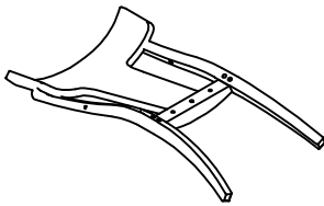
x1 RP306DJ261-BACK-Chair back Dossier de chaise Respaldo de la silla
